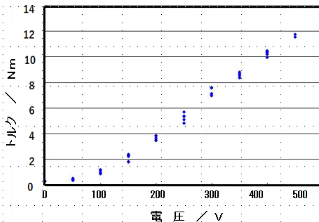
図 多重シリンダ型ER流体ブレーキのトルク性能
